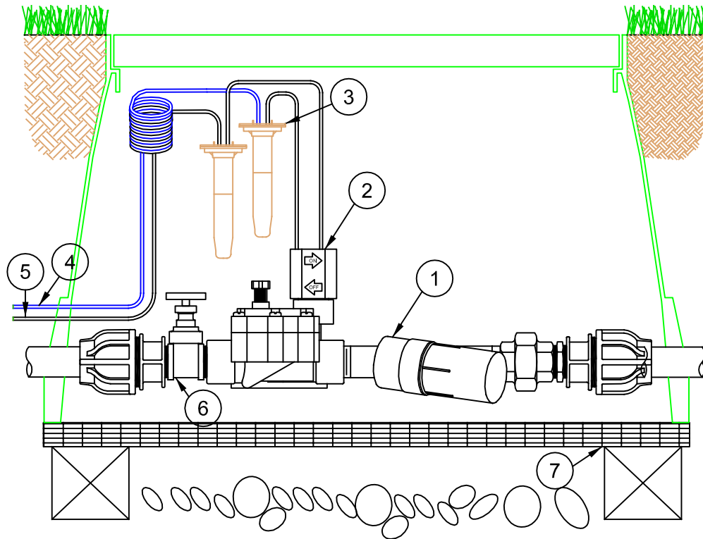
Filter- und Regeleinheit X CZ-075-PRF
