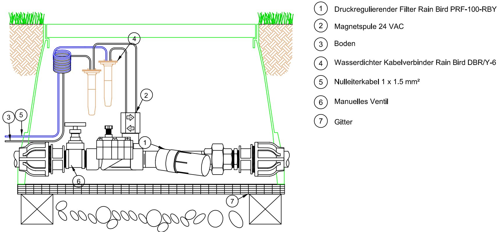
Filter- und Regeleinheit X CZ-100-PRF
